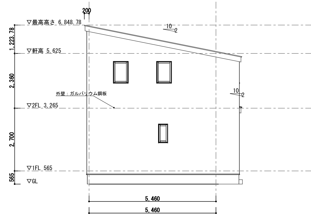
東立面図
