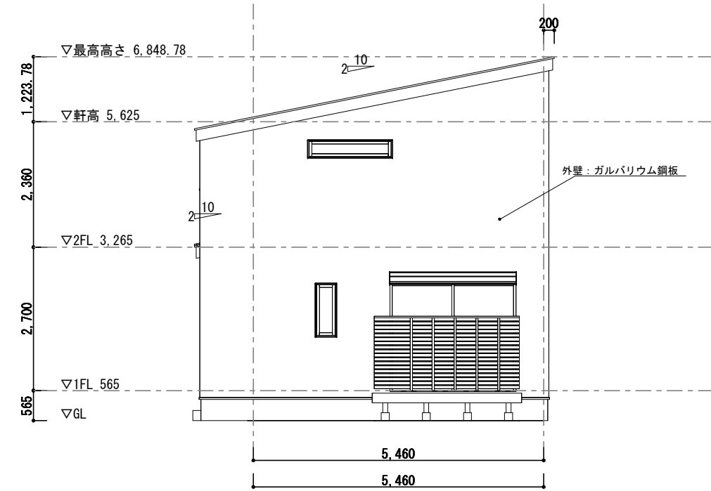
東立面図
