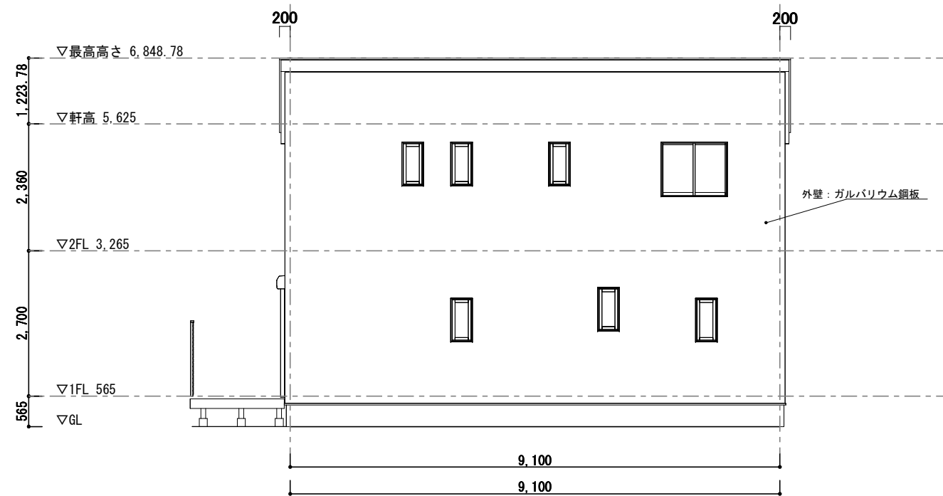
南立面図
