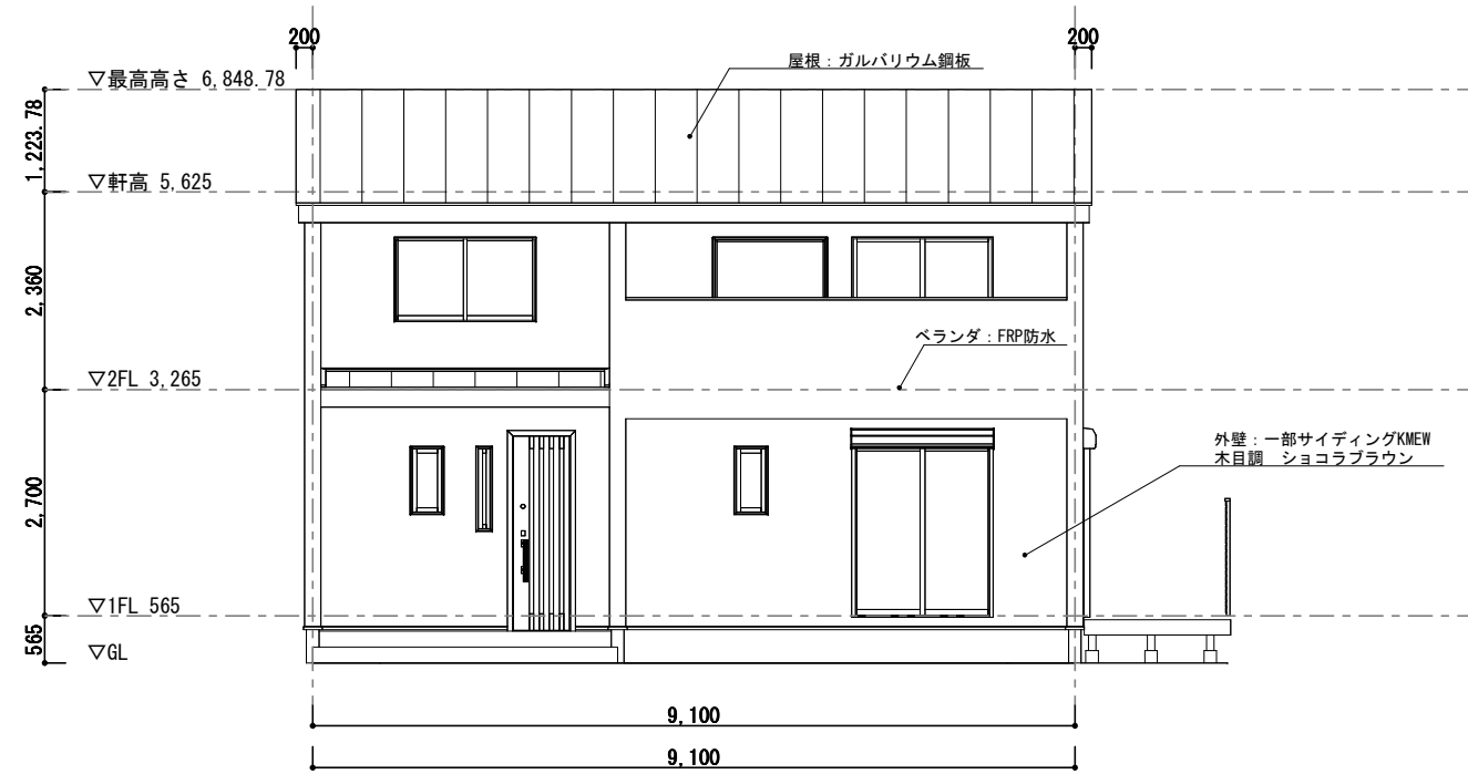
南立面図
